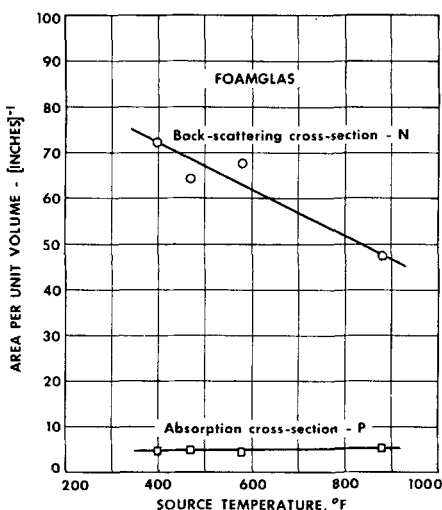
Fig. 6. Radiation parameters for Foamglas.
