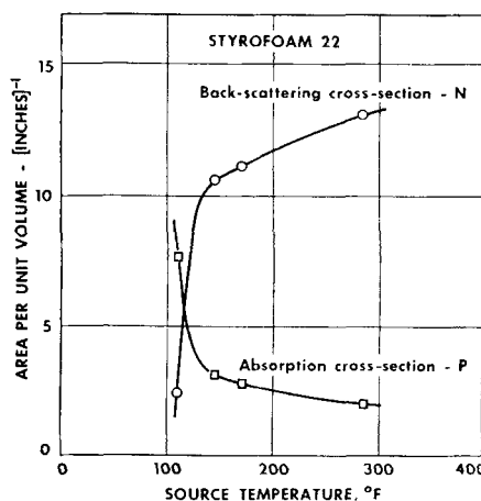
Fig. 7. Radiation parameters for Styrofoam-22.
